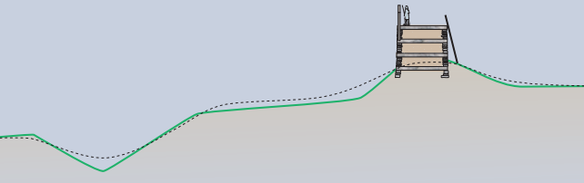
Schematisches Profil durch den Keltenwall mit Ergänzung des ursprünglichen Zustandes.
